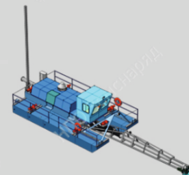
Земснаряд Д-110/47-И-1 970 м 3 в час / 56 м.вод.ст.
