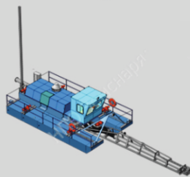
Земснаряд Д-110/47-И-2-2 1780 м 3 в час / 31 м.вод.ст.
